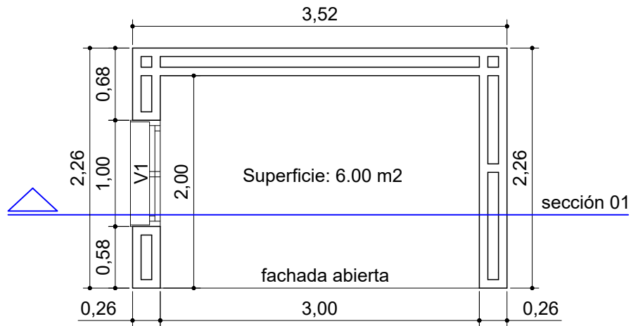
PLANTA DISTRIBUCION
